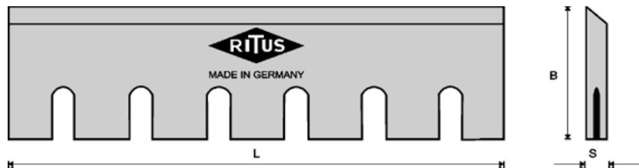
L = Länge/length x B = Breite/width x S = Stärke/thickness in mm
